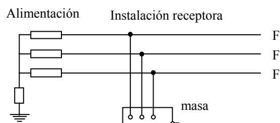
Esquema IT
