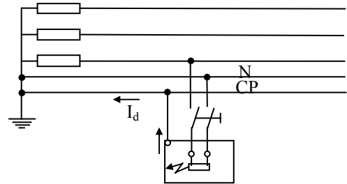
Esquema TN-S
