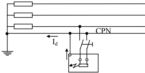
Esquema TN-C
